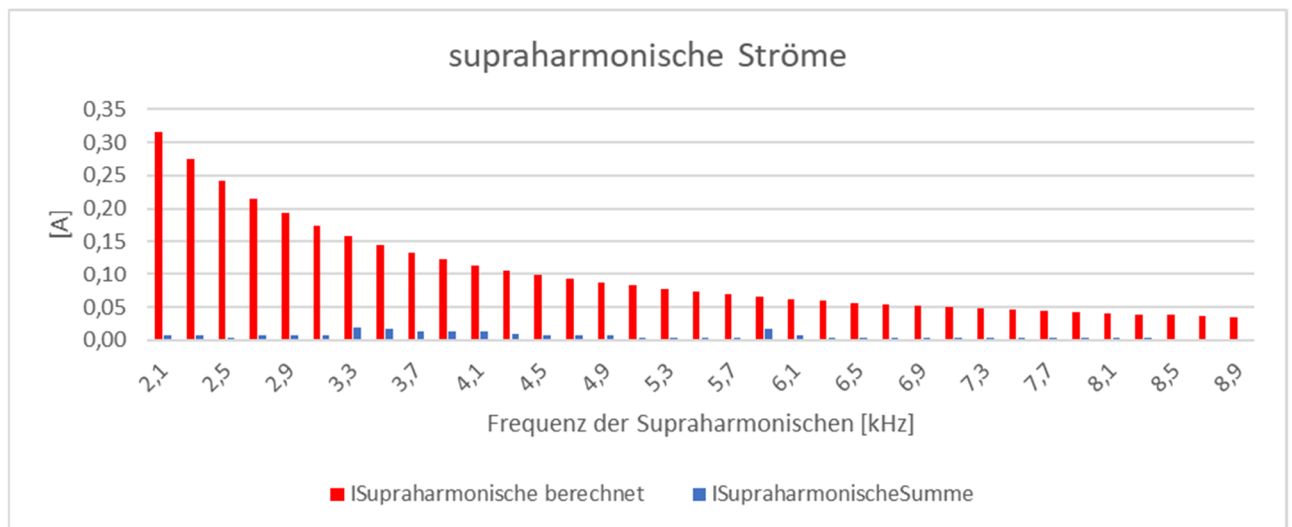
Bild 4: Zulässige und höchste supraharmonische Ströme der EZA
