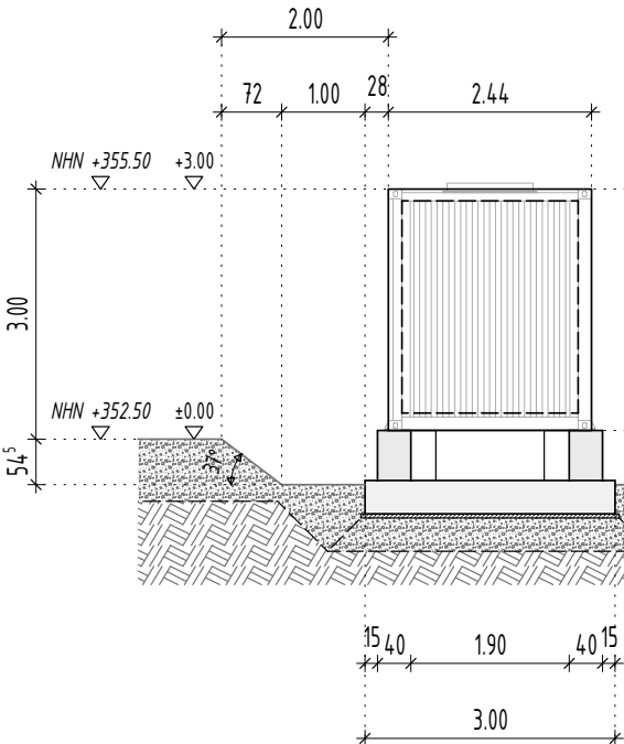
SCHNITT / ANSICHT quer
